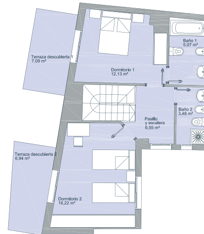
PLANTA BAJOCUBIERTA
